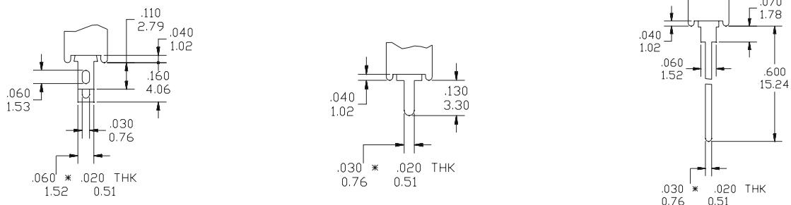
M1 Solder
